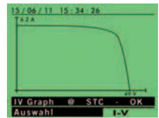
Grafische Darstellung der gemessenen I-U Kennlinie
