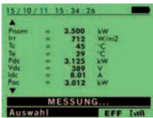
Messung / Aufzeichnung in der Funktion Leistungsanalyse
