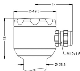
Kompakt-Feldgehäuse (IP 67)
