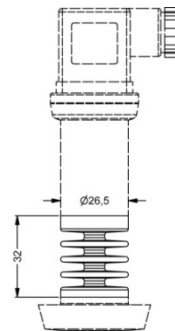
Temperatorkoppler 300 °C
