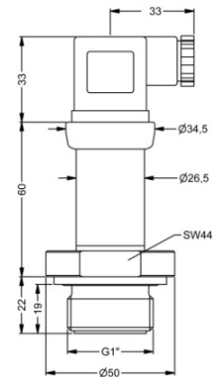
G1" frontbündig DIN 3852 mit ISO 4400
