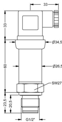
G1/2" frontbündig mit radialem O-Ring 9
