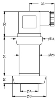
Milchröhr (DIN 11851) mit ISO 4400
